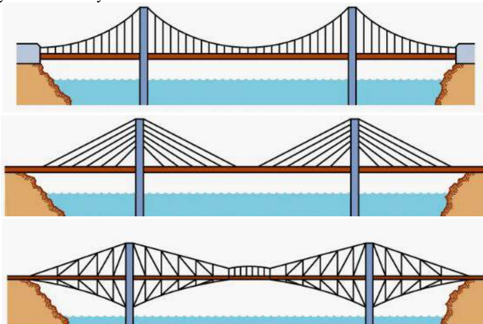
1-rasm. O'sma, vantli va kombinatsiyalangan oraliq qurilmalar
